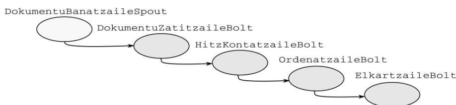
5.10 irudia: Gehien agertu diren hitzak ordenatuta zerrendatzeko adibidearen Storm topologia lineala.
